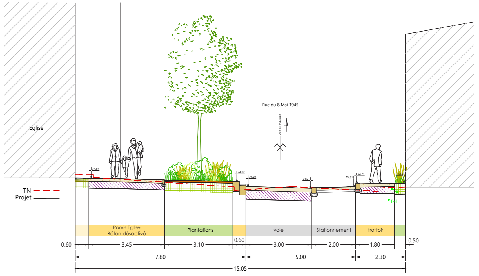
Coupe Projet
