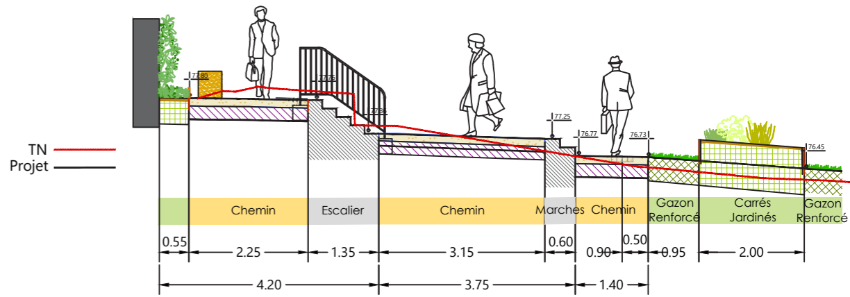
Coupe Projet
