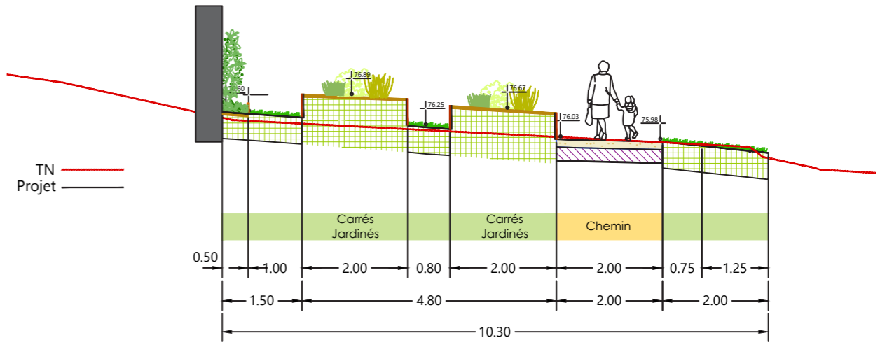
Coupe Projet
